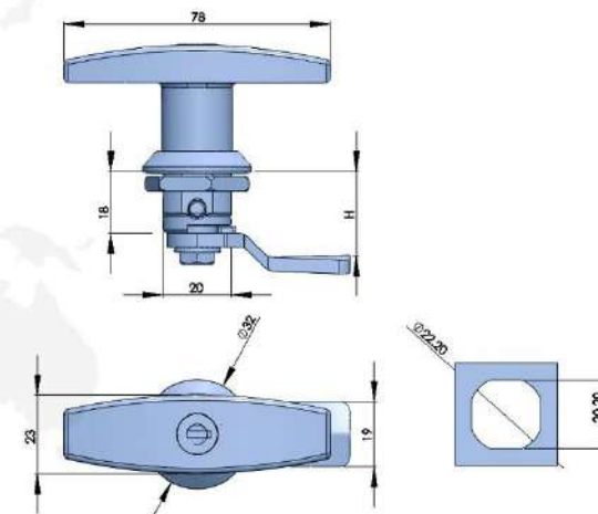
316不锈钢T型把手 T-HANDLE AISI 316
