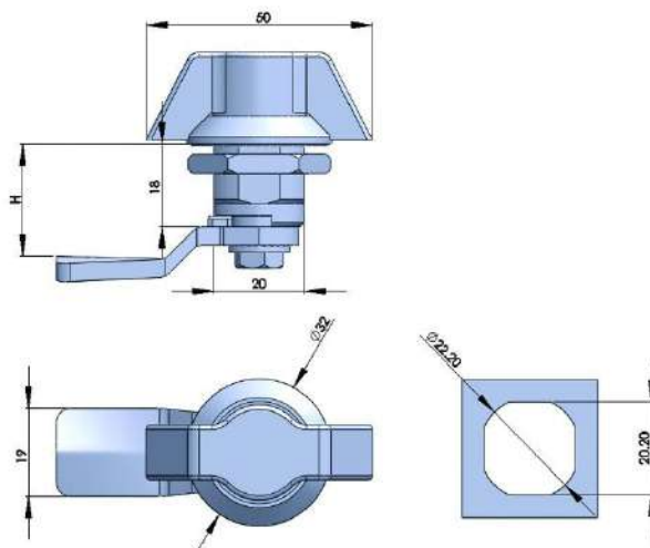
316不锈钢把手 WING KNOB AISI316
