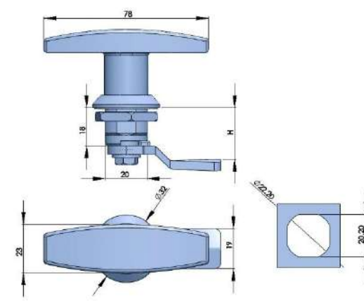
316不锈钢T型把手 T-HANDLE AISI 316
