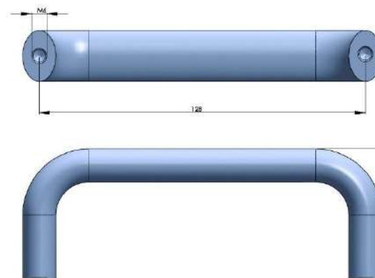
把手 HANDLE 2310-0115-B5
