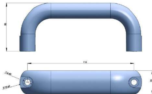
316不锈钢把手 HANDLE AISI 316
