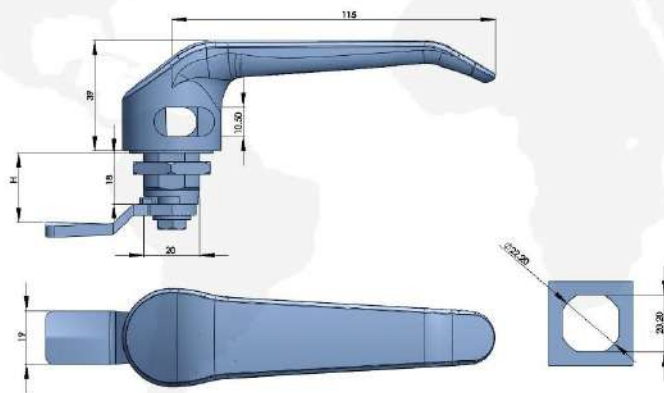
316不锈钢挂锁把手 L-HANDLE FOR PADLOCK AISI 316
