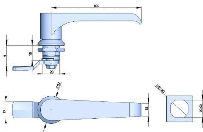
316不锈钢L型把手 L-HANDLE AISI 316
