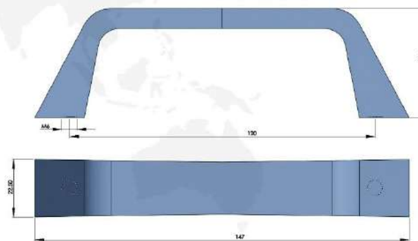
316不锈钢把手 HANDLE AISI 316
