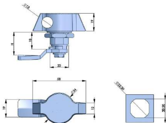
把手 FOR PADLOCK 2310-0117-B5
