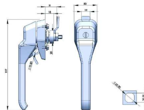
316不锈钢把手 HEAVY DUTY HANDLE AISI316
