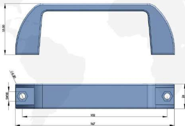
316不锈钢把手 HANDLE AISI 316
