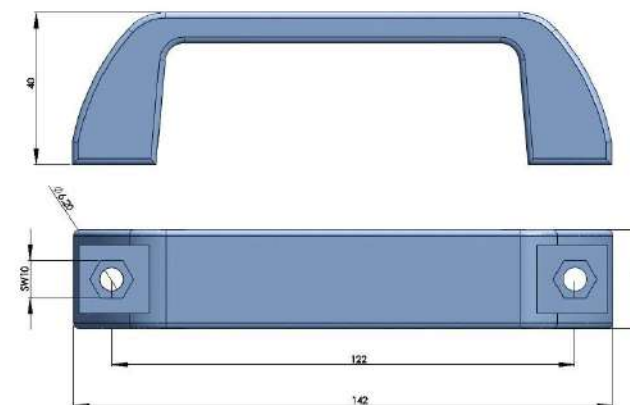
316不锈钢把手 HANDLE AISI 316
