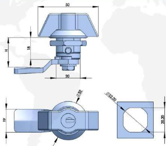
316不锈钢把手 WING KNOB AISI316
