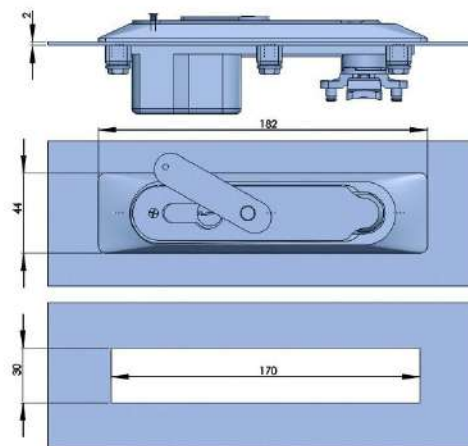
316不锈钢手柄 SWINGHANDLE AISI316
