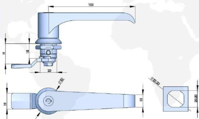
316不锈钢L型把手 L-HANDLE AISI 316
