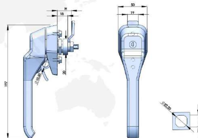
316不锈钢把手 HEAVY DUTY HANDLE AISI316
