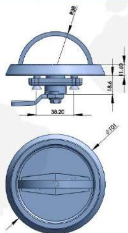
把手 HANDLE 2310-0116-B5
