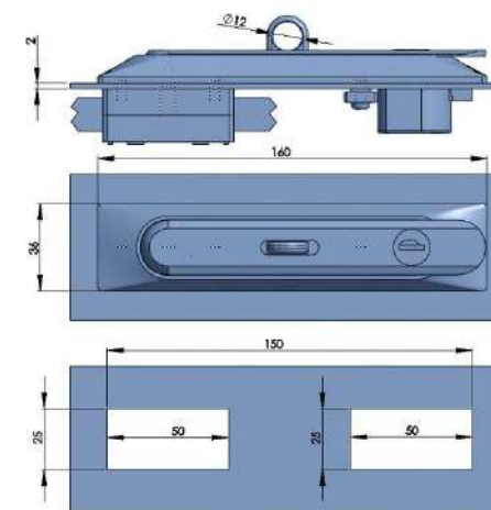
316不锈钢手柄 SWINGHANDLE AISI316
