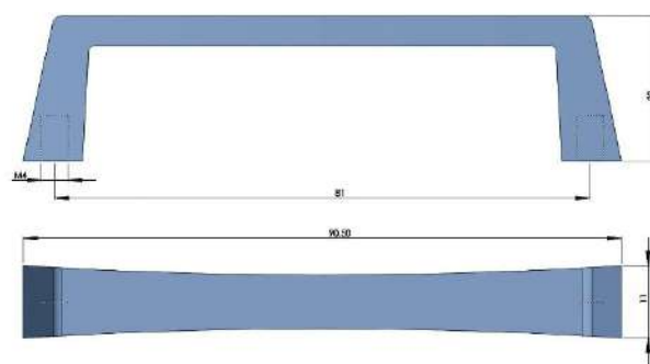
316不锈钢把手 HANDLE AISI 316
