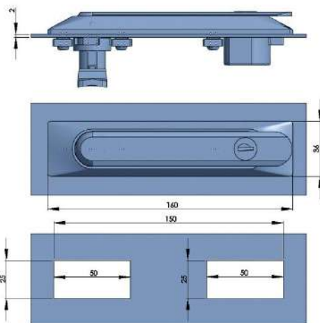
316不锈钢手柄 SWINGHANDLE AISI316
