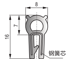
MF-015 黑色三元乙丙钢丝胶条 Black EPDM steel wire strip
