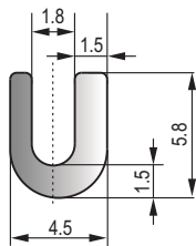
MFT-073 黑色三元乙丙密实胶条 Black EPDM Dense Strip
