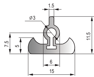
MFT-066 黑色三元乙丙密实胶条 Black EPDM Dense Strip
