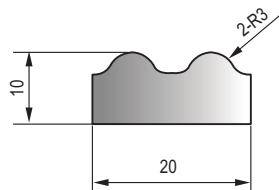
MFT-038 黑色三元乙丙海绵胶条 Black EPDM Sponge Strip
