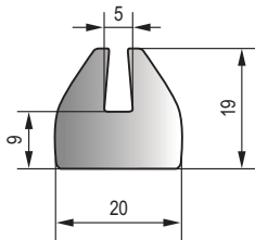
MFT-077 黑色三元乙丙密实胶条 Black EPDM Dense Strip
