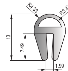
MFT-056 黑色三元乙丙密实胶条 Black EPDM Dense Strip
