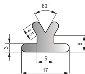
MFT-053 黑色三元乙丙海绵胶条 Black EPDM Sponge Strip
