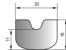
MFT-032 黑色三元乙丙海绵胶条 Black EPDM Sponge Strip
