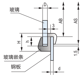
MFT-062 黑色三元乙丙密实胶条 Black EPDM Dense Strip
