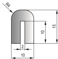
MFT-027 黑色三元乙丙海绵胶条 Black EPDM Sponge Strip
