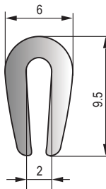
MFT-076 黑色三元乙丙密实胶条 Black EPDM Dense Strip
