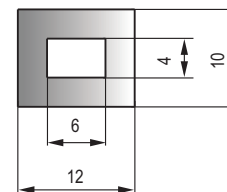
MFT-034 黑色三元乙丙海绵胶条 Black EPDM Sponge Strip
