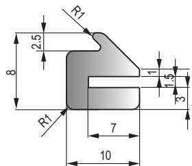
MFT-028 黑色三元乙丙海绵胶条 Black EPDM Sponge Strip
