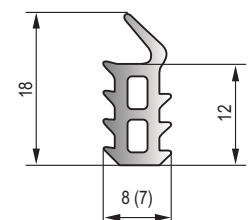
MFT-060 黑色三元乙丙密实胶条 Black EPDM Dense Strip
