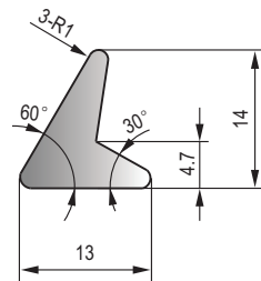
MFT-029 黑色三元乙丙海绵胶条 Black EPDM Sponge Strip
