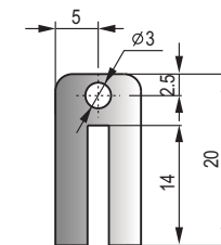
MFT-035 黑色三元乙丙海绵胶条 Black EPDM Sponge Strip
