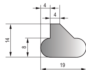
MFT-033 黑色三元乙丙海绵胶条 Black EPDM Sponge Strip
