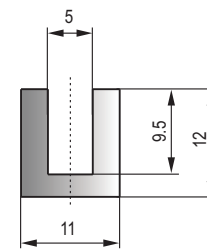
MFT-071 黑色三元乙丙密实胶条 Black EPDM Dense Strip
