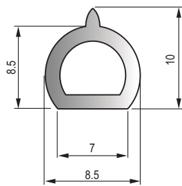
MFT-065 PVC密封胶条 PVC gasketing
