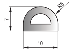
MFT-048 黑色三元乙丙海绵胶条 Black EPDM Sponge Strip
