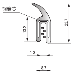
MF-013 黑色三元乙丙钢丝胶条 Black EPDM steel wire strip
