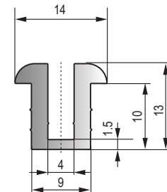
MFT-072 黑色三元乙丙密实胶条 Black EPDM Dense Strip
