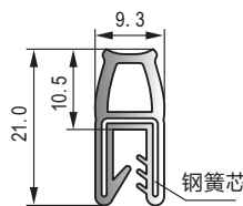
MF-017 黑色三元乙丙钢丝胶条 Black EPDM steel wire strip
