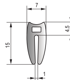
MFT-058 黑色三元乙丙密实胶条 Black EPDM Dense Strip
