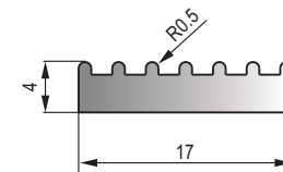
MFT-047 黑色三元乙丙海绵胶条 Black EPDM Sponge Strip
