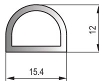
MFT-050 黑色三元乙丙海绵胶条 Black EPDM Sponge Strip
