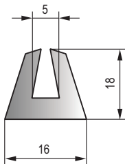
MFT-078 黑色三元乙丙密实胶条 Black EPDM Dense Strip
