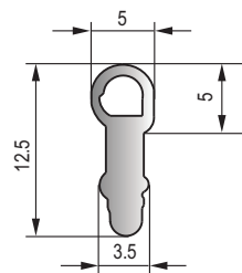
MFT-041 黑色三元乙丙海绵胶条 Black EPDM Sponge Strip
