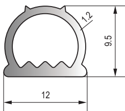
MFT-040 黑色三元乙丙海绵胶条 Black EPDM Sponge Strip
