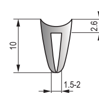
MFT-059 黑色三元乙丙密实胶条 Black EPDM Dense Strip
