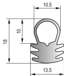
MFT-016 黑色三元乙丙密实发泡密封条 Black EPDM sealing strip
