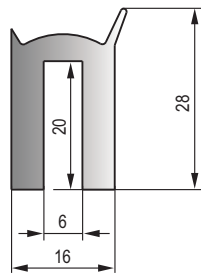
MFT-075 黑色三元乙丙密实胶条 Black EPDM Dense Strip
