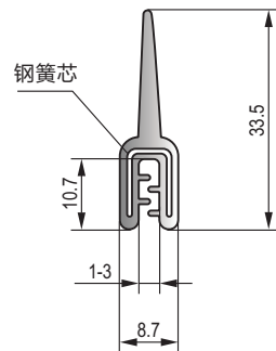
MF-014 黑色三元乙丙钢丝胶条 Black EPDM steel wire strip
