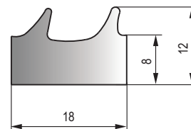
MFT-051 黑色三元乙丙海绵胶条 Black EPDM Sponge Strip
