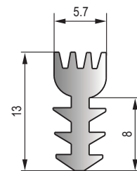
MFT-030 黑色三元乙丙海绵胶条 Black EPDM Sponge Strip
