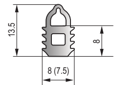
MFT-061 黑色三元乙丙密实胶条 Black EPDM Dense Strip
