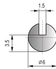
MFT-070 黑色三元乙丙密实胶条 Black EPDM Dense Strip
