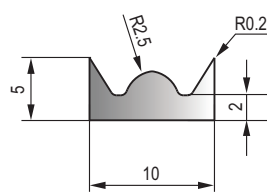
MFT-026 黑色三元乙丙海绵胶条 Black EPDM Sponge Strip
