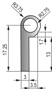
MFT-074 黑色三元乙丙密实胶条 Black EPDM Dense Strip
