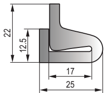
MFT-037 黑色三元乙丙海绵胶条 Black EPDM Sponge Strip
