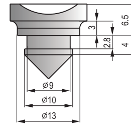
MFT-044 EPDM门用缓冲钉 EPDM door nail buffer
