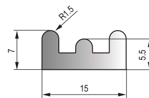
MFT-046 黑色三元乙丙海绵胶条 Black EPDM Sponge Strip
