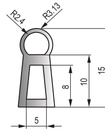
MFT-031 黑色三元乙丙海绵胶条 Black EPDM Sponge Strip
