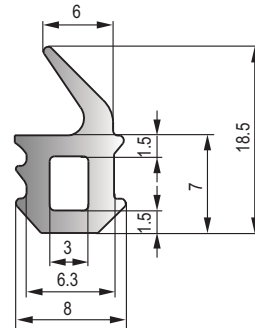
MFT-067 黑色三元乙丙密实胶条 Black EPDM Dense Strip
