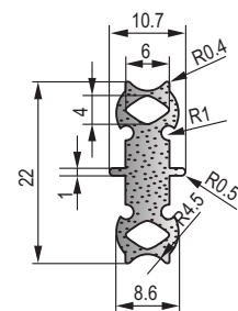
MFT-052 黑色三元乙丙海绵胶条 Black EPDM Sponge Strip
