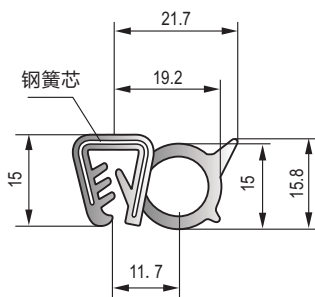
MF-016 黑色三元乙丙钢丝胶条 Black EPDM steel wire strip
