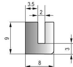
MFT-069 黑色三元乙丙密实胶条 Black EPDM Dense Strip
